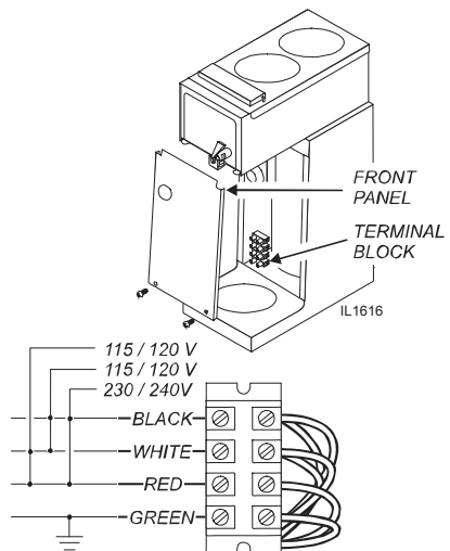
Fig. 3 115/240 Volt Terminal Block
